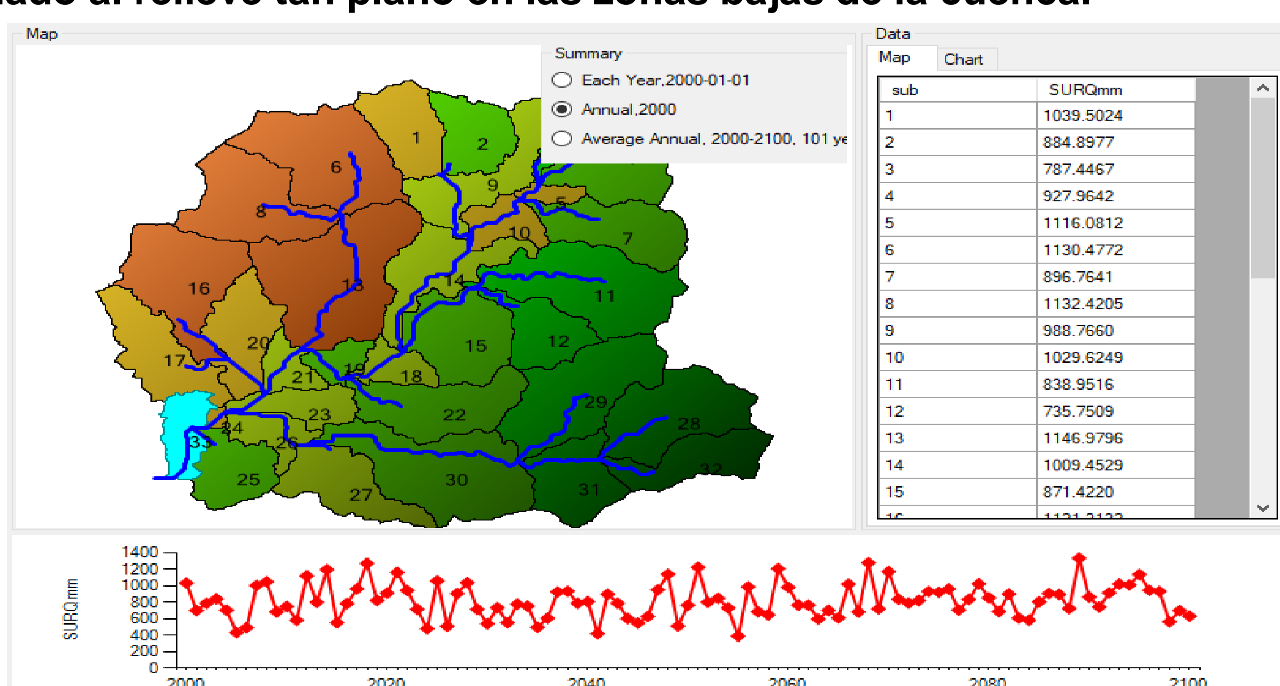
Figura 2: Lámina de escorrentía (mm) periodo 2000 - 2100 del modelo hidrológico generado por SWAT del Acuífero Huacas Tamarindo, Santa Cruz, Guanacaste.
