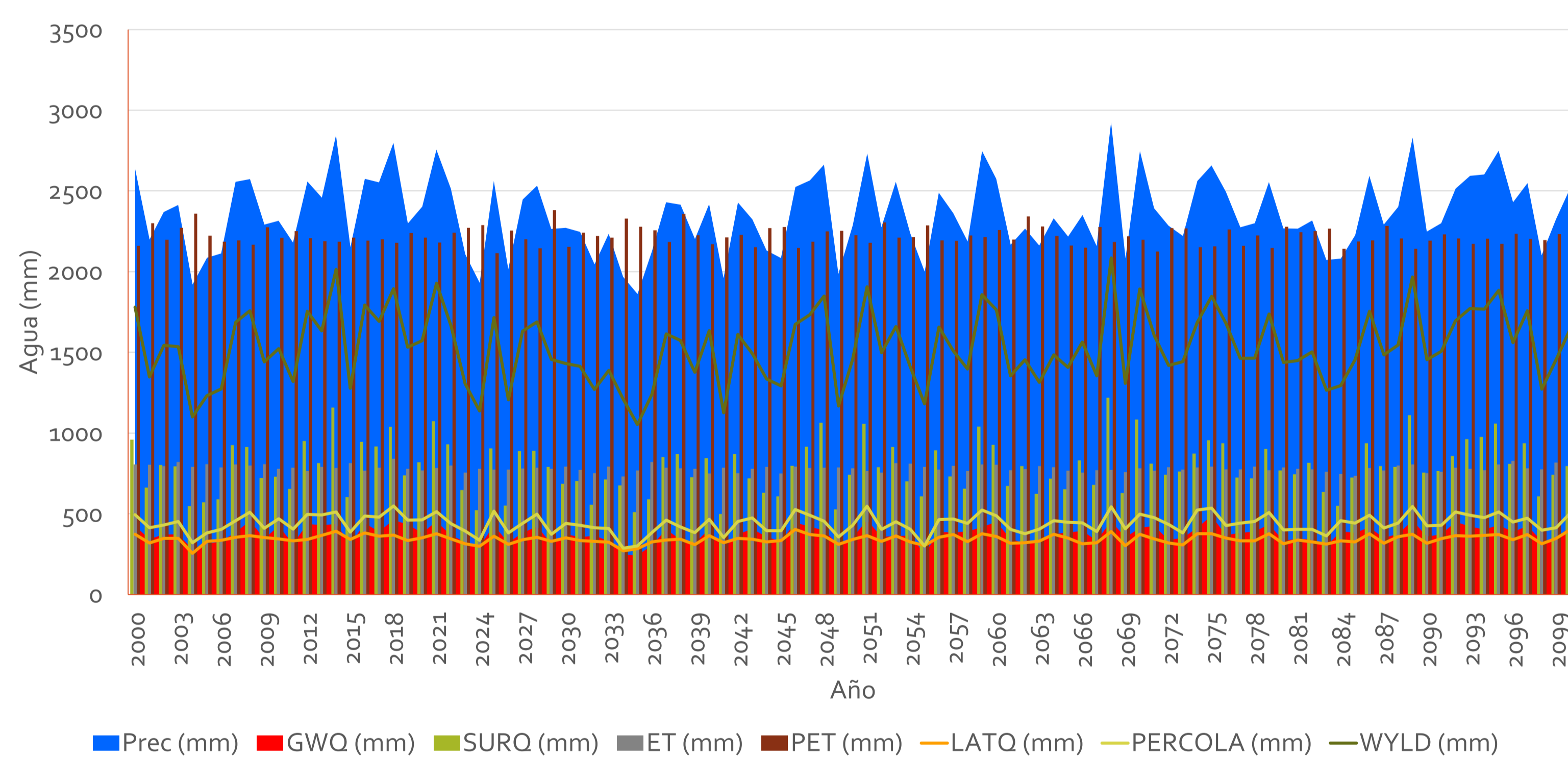
Nota: PREC= precipitación. SURQ= Escorrentía superficial. LATQ= Flujo lateral. GWQ= Agua subterránea. PERCOLA= Percolación. ET= Evapotranspiración. PET= Evapotranspiración potencial. WYLD= Rendimiento del agua.
